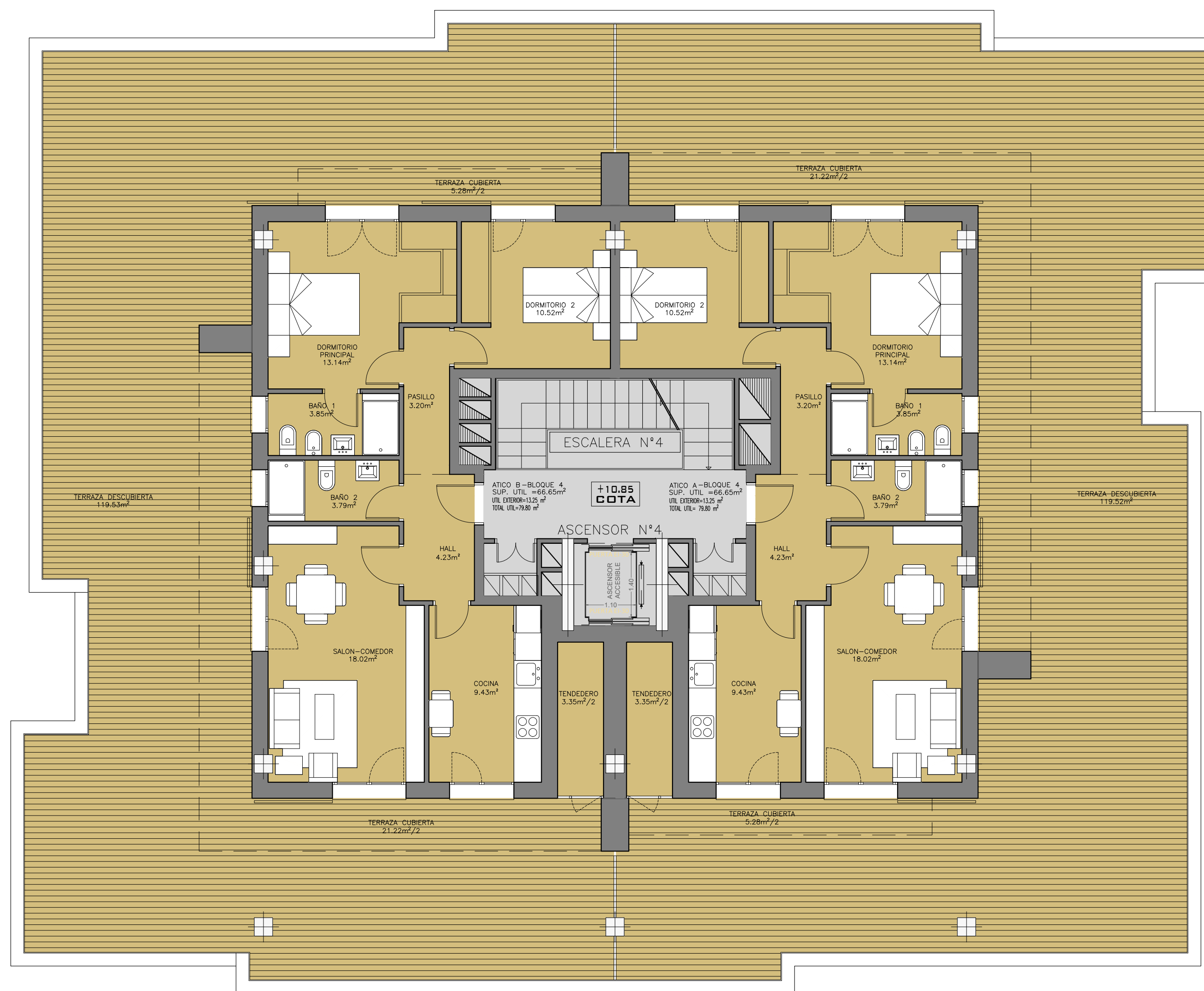
PLANTA ATICO BLOQUE B4
