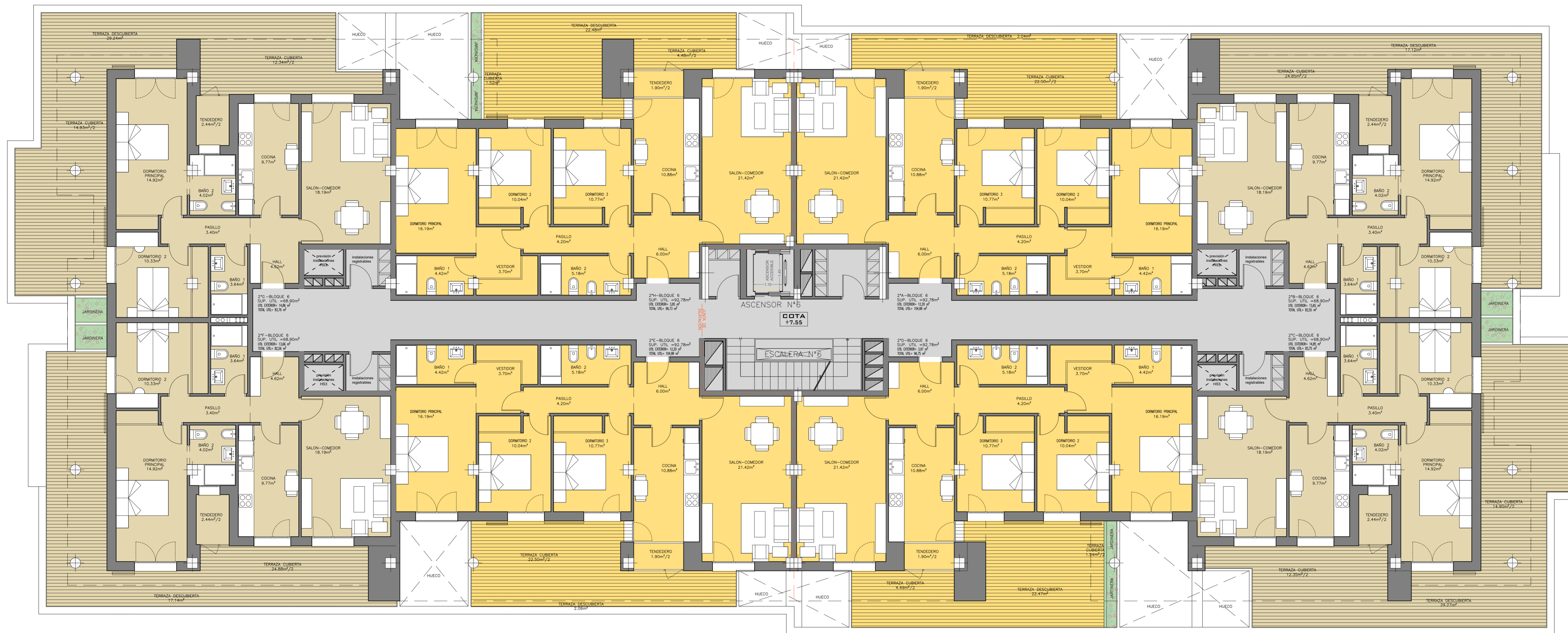
PLANTA SEGUNDA BLOQUE B6
